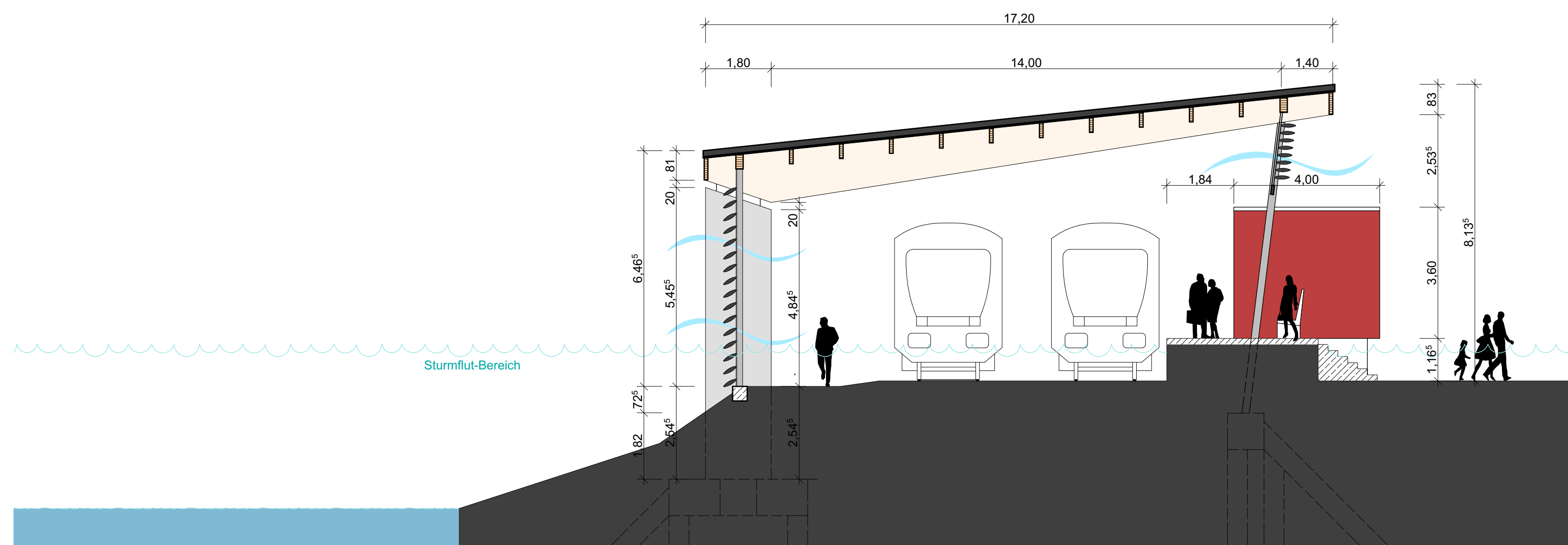
Querschnitt_M. 1:100
